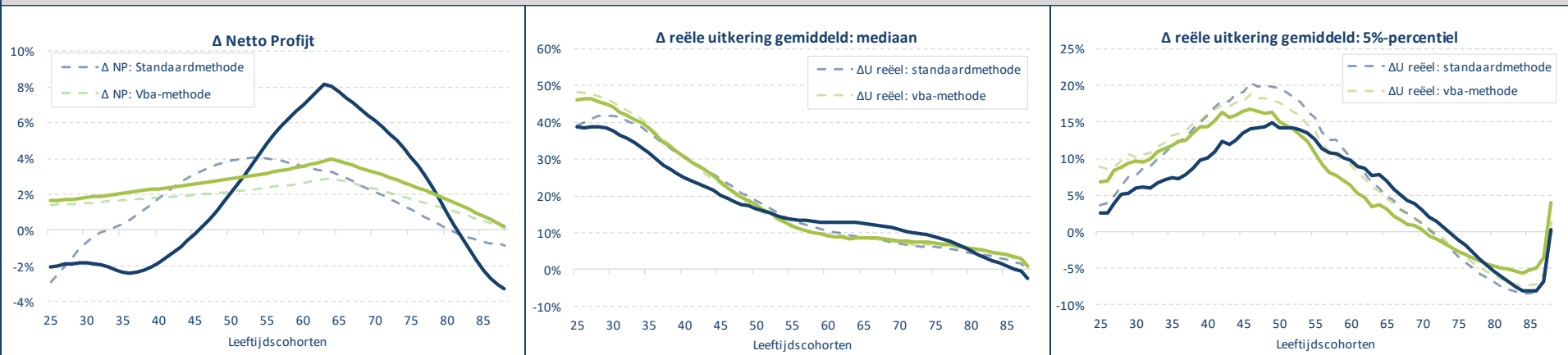
renteschok -100bps
