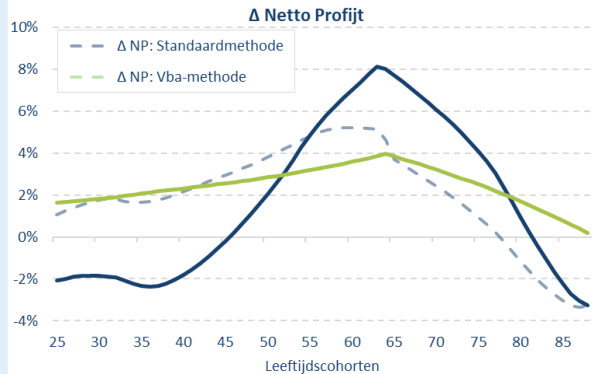
Basis dekkingsgraad 122%
