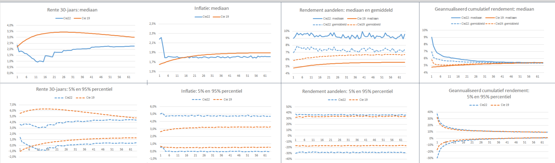
Scenario's P
