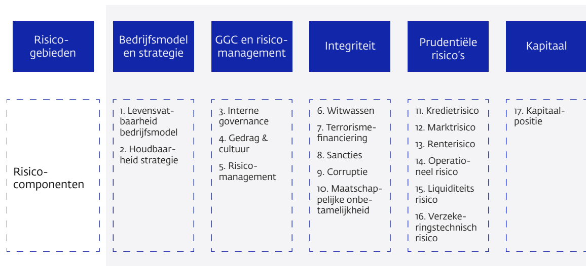
Figuur 2 Risicotaxonomie*
